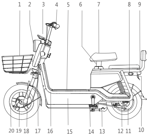
整车结构示意图
