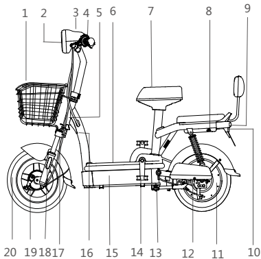
整车结构示意图
