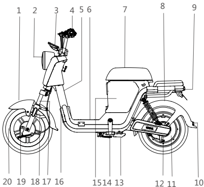
整车结构示意图
