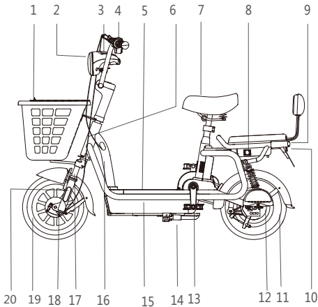
整车结构示意图
