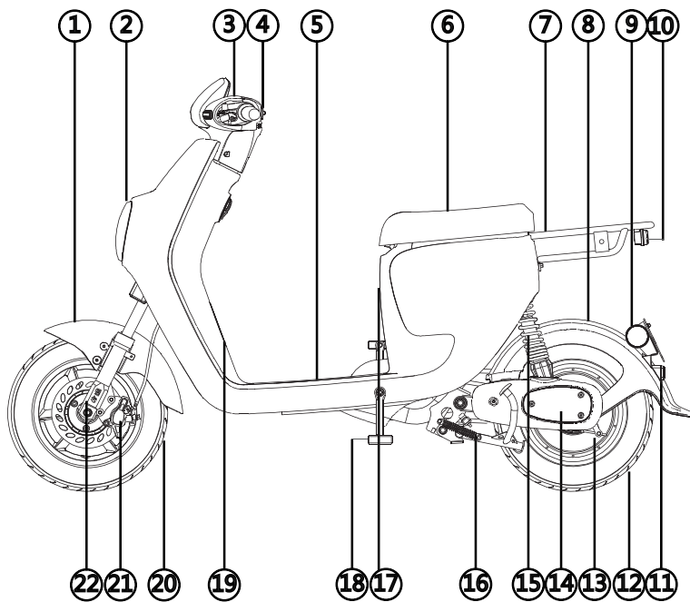
整车结构示意图
